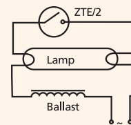
SINGLE 220-240 V~
