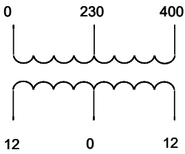
Egyfázisú biztonsági transzformátorok Primer feszültség 230, 400V. Szekunder feszültség 24V (12V-0-12V). Hőállósági osztály B
